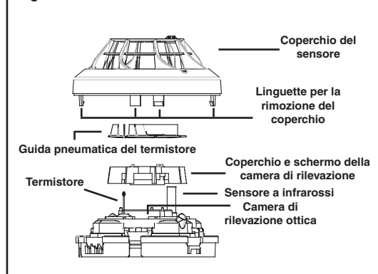
Figura 2: Pulizia del sensore
