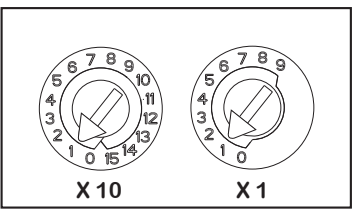
Abbildung 1: Drehschalter für die Adressierung
