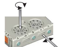
FIGURA 4: CONEXIONES DEL MÓDULO DE ENTRADA DOBLE Y SALIDA ÚNICA M221E
