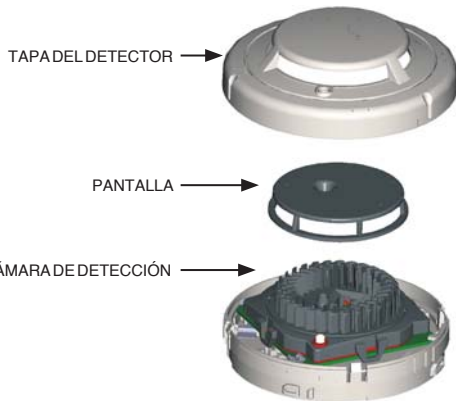
Figura 3: Detector Óptico de Humo 2351E
