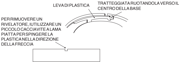
Figura 3: Rivelatore Ottico di Fumo 2351E
