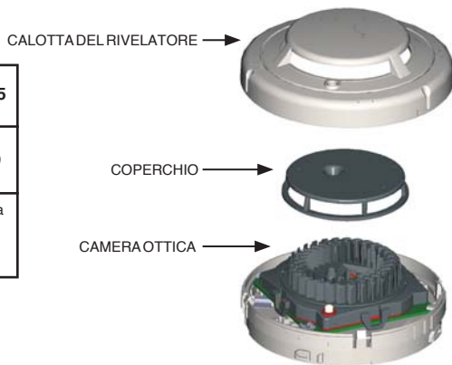
Figura 3: Rivelatore Ottico di Fumo 2351E
