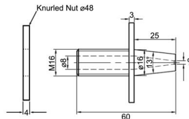
FAAST-PIPESPKIT FAAST Sampling Point Kit
