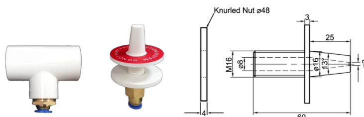
FAAST-PIPESPKIT FAAST Sampling Point Kit
