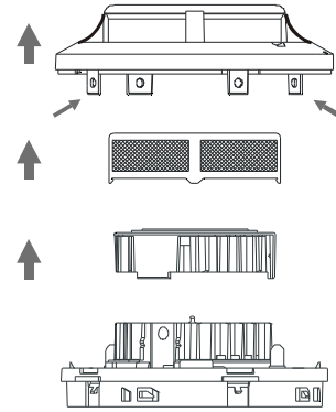
Abb.1: Reinigung des Rauchmelders
